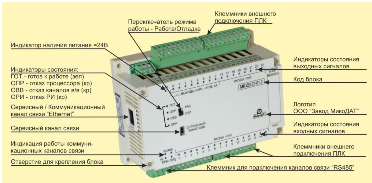
Структурная схема ПЛК МК120
