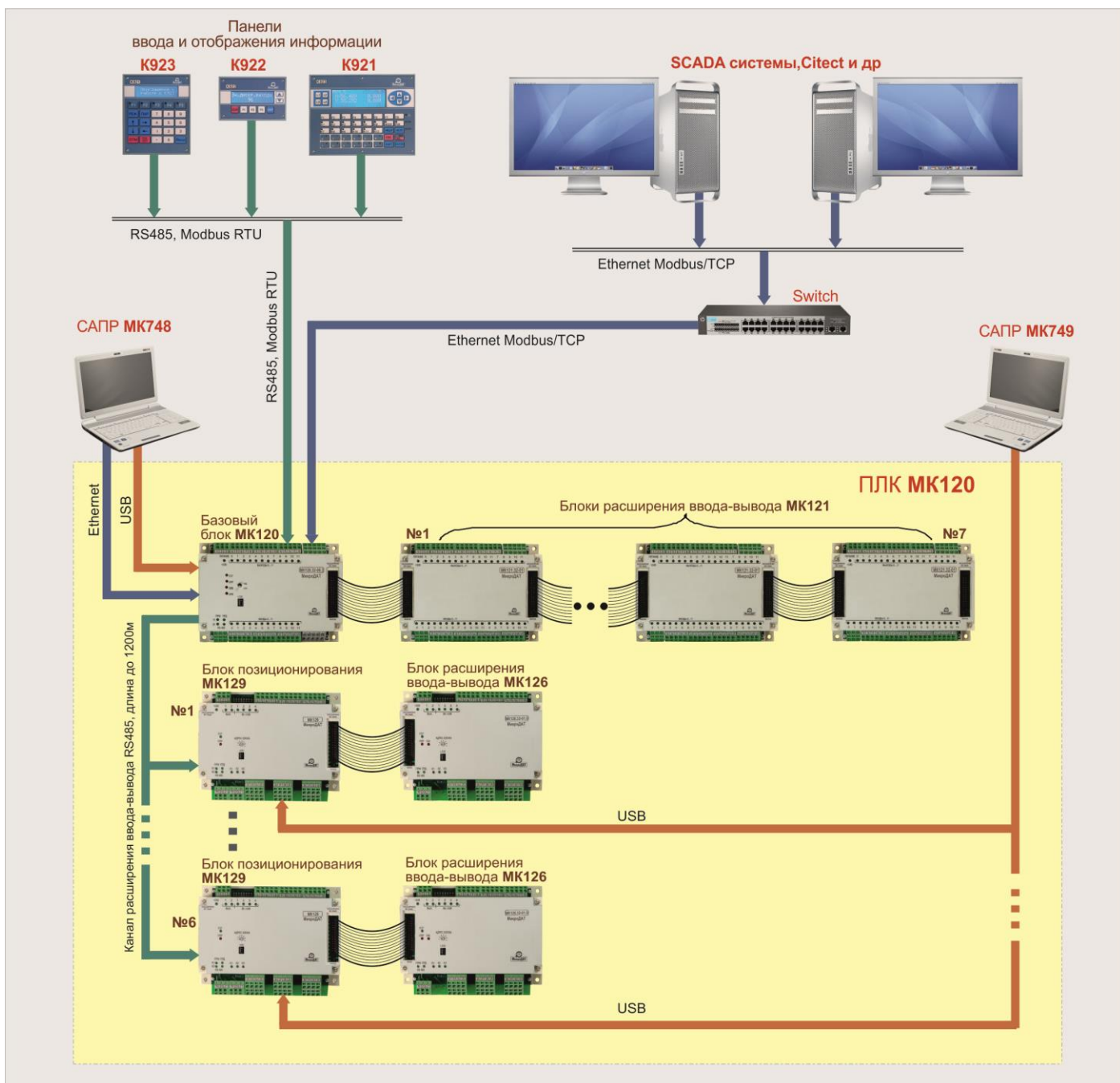
Структурная схема ПЛК МК120
